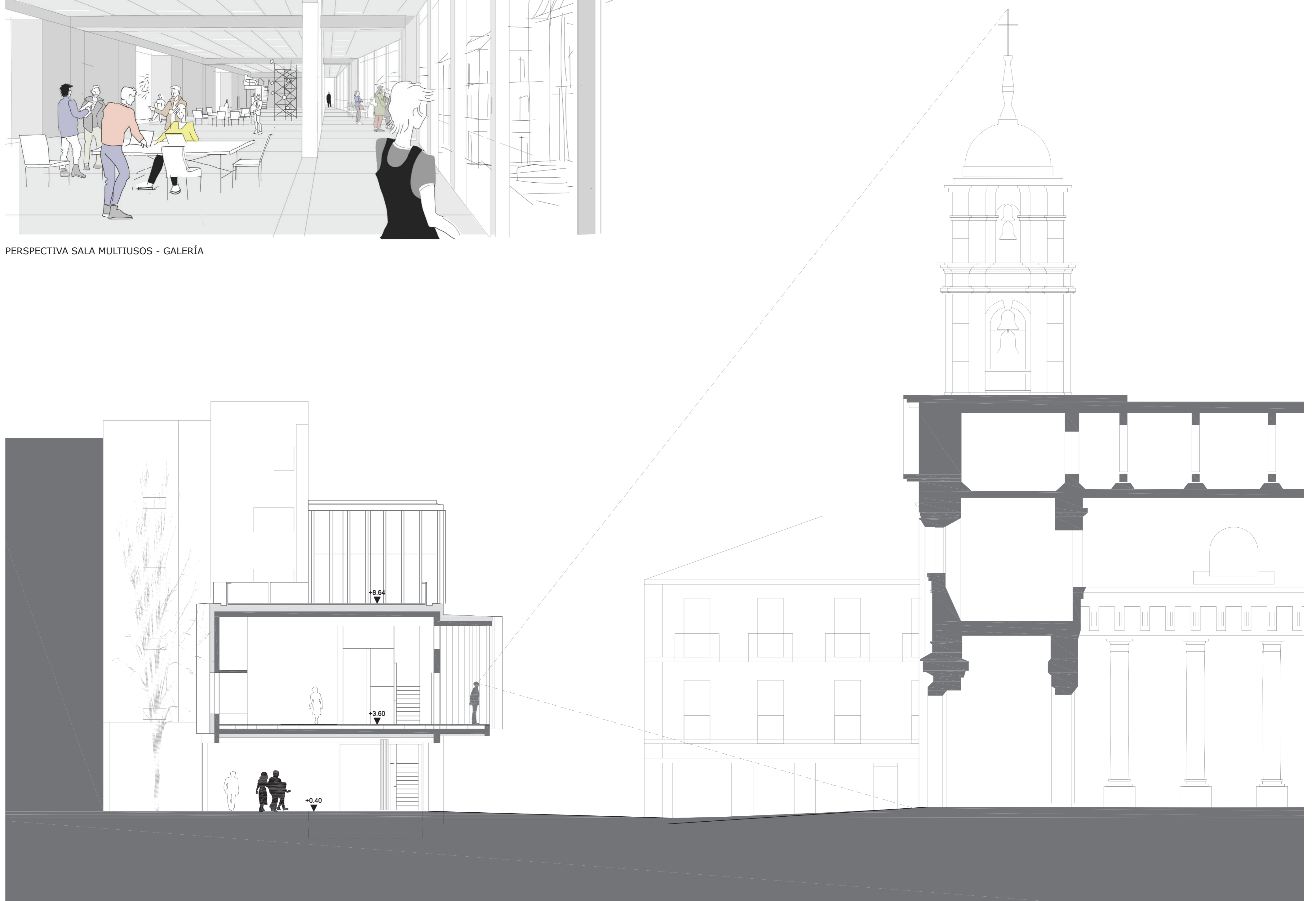
SECCIÓN TRANSVERSAL. ESPACIOS PÚBLICOS USOS MÚLTIPLES EN TRES NIVELES, PLANTA BAJA_PLAZA, PRIMERA Y CUBIERTA. Esc 1:200
