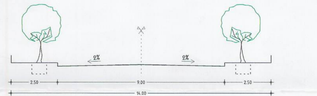
PERFIL TIPO CAMINO DE GOALDINO
