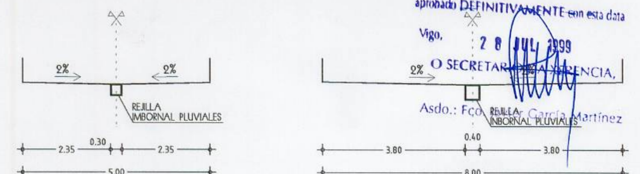
PERFIL TIPO RUAS MIXTAS AREAS CONSOLIDADAS
