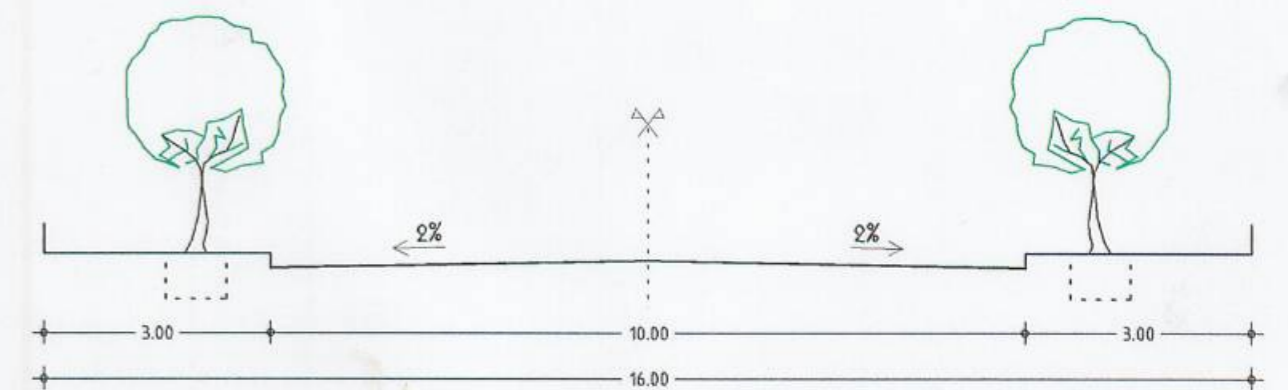
PERFIL TIPO ESTRADA DE PORTO
