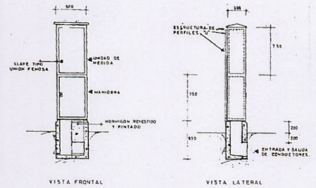
VISTA FRONTAL VISTA LATERAL CUADRO DE MANDA, PROTECCION Y MANIOBRA EJ 1/20
