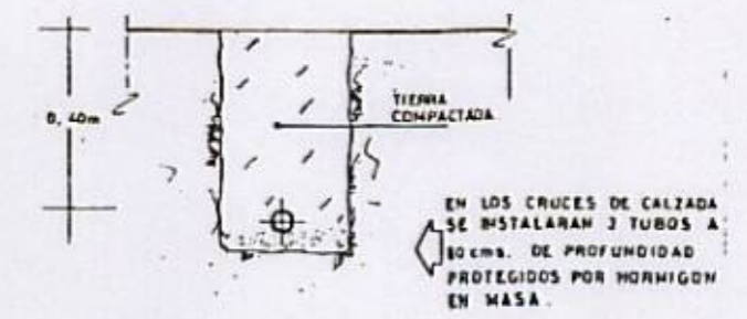
SECCION DE ZANJA.
