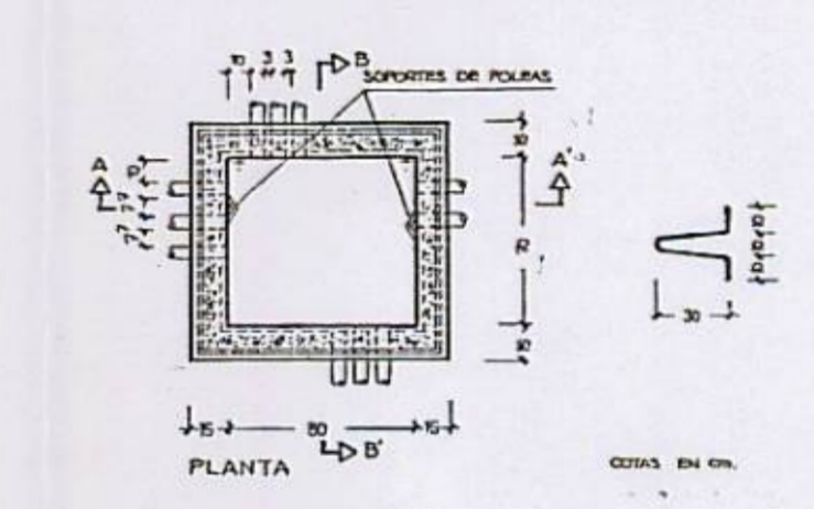
Arqueta tipo "M"
