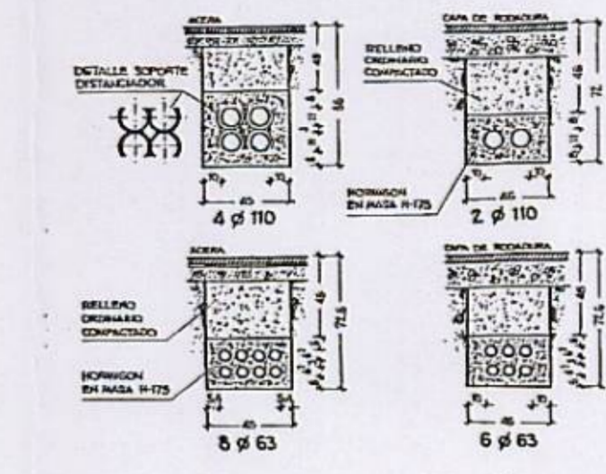
Secciones tipo de zanjas
