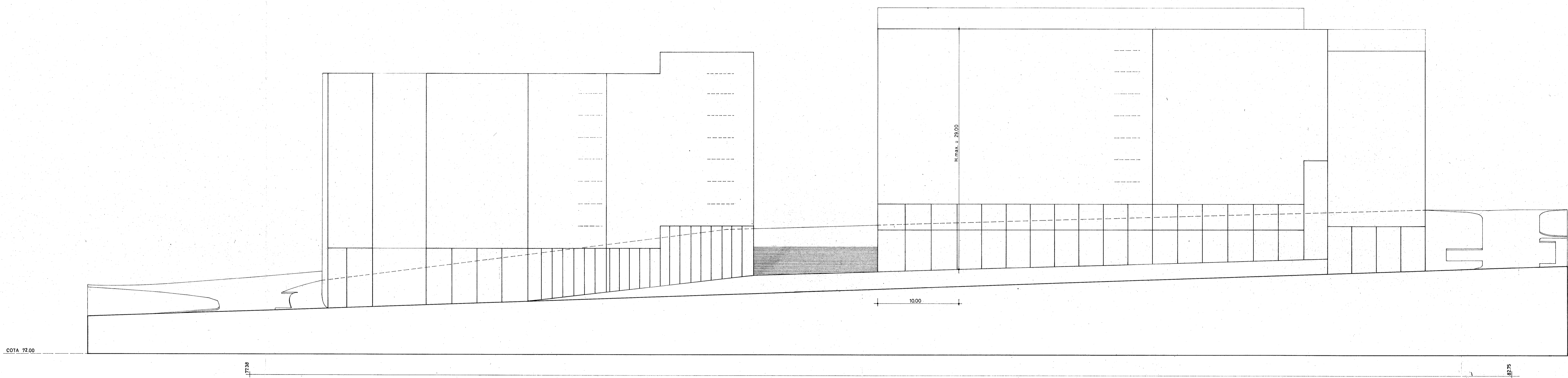
ALZADO-SECCION C/GREGORIO ESPINO E 1/200
