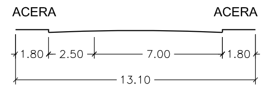
SECCION V-3 (ZONA P-2)
