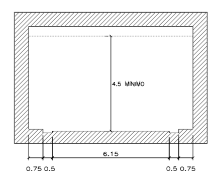
SECCIÓN TIPO TUNEL E:1/200
