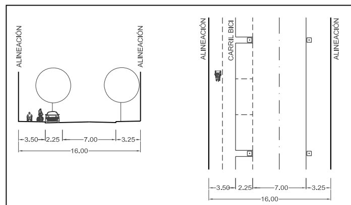
SECCION TIPO CALLE 16 m.
