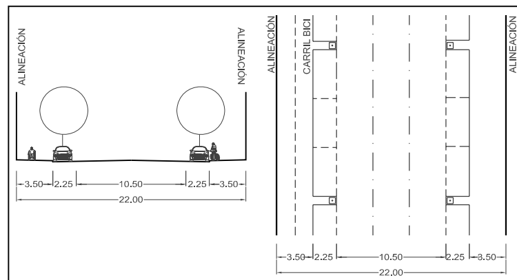
SECCION TIPO CALLE 22 m.
