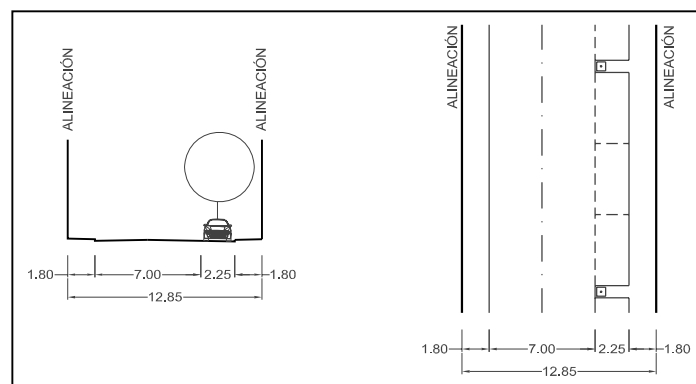
SECCION TIPO RUA SANTA CRISTINA
