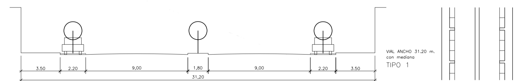
SECCIÓN DE VIALES. Esc. 1 : 200
