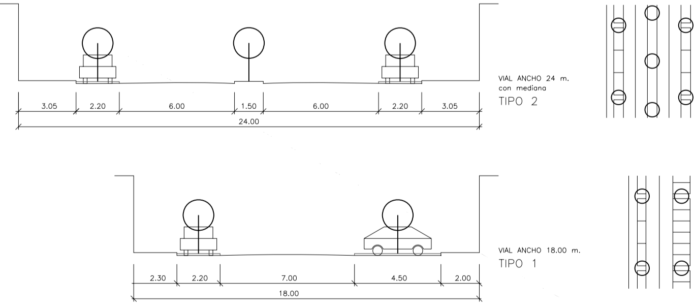
SECCIÓN DE VIAES. Esc. 1 : 200
