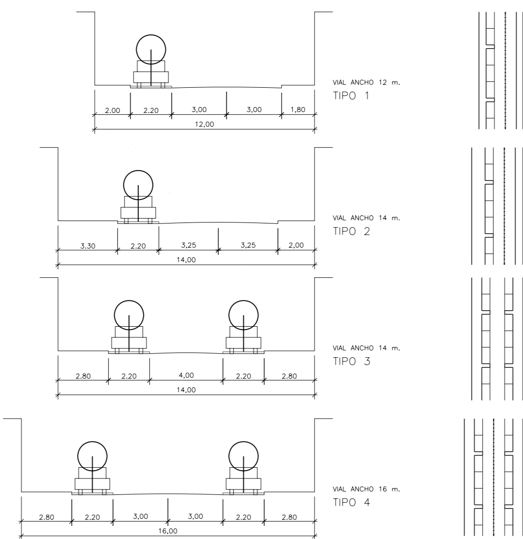
SECCIÓN DE VIALES. Esc. 1:200
