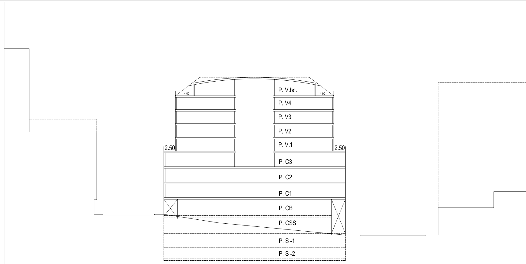
SECCIÓN CORTE A-A ESCALA 1/500
